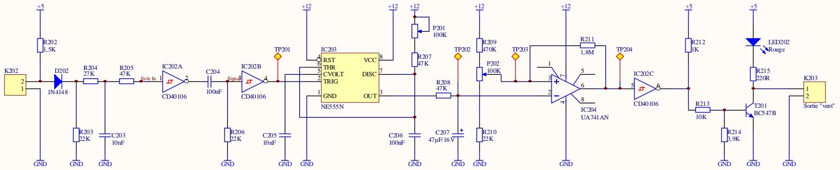
Capteur éolien (4 pulses/tour)
